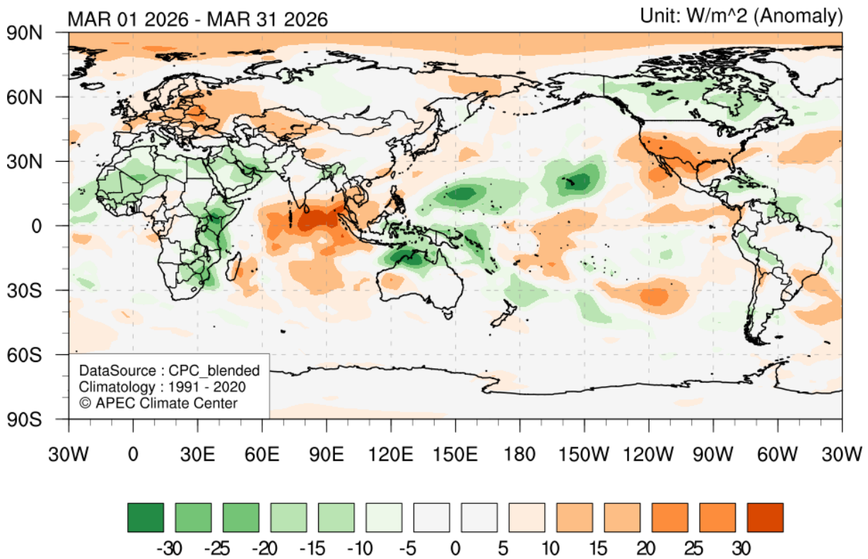
2026 3월 기온 (위) 및 상향장파복사(아래)의 평년대비 편차 (평년 : 1991-2020)
