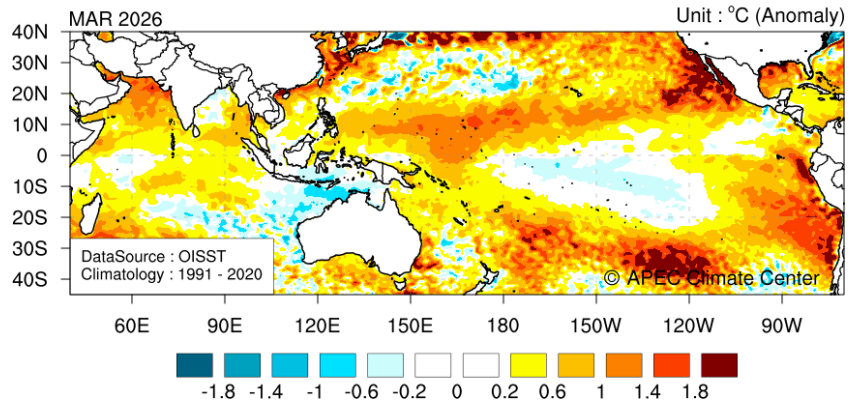
2026 3월 해수면 온도 분포(위) 및 평년대비 편차(아래) (평년: 1991-2020)
