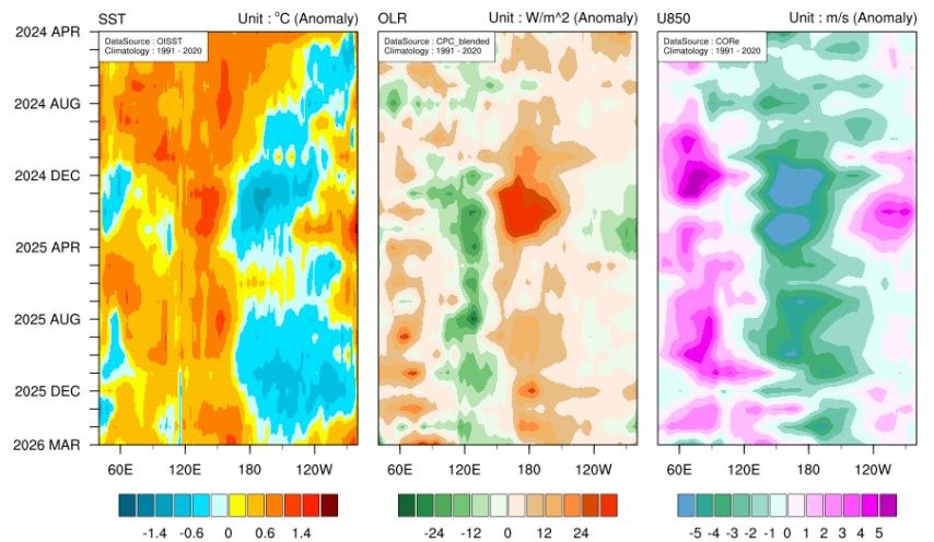
2024 4월 - 2026 3월 적도지역 해수면온도, 상향장파복사, 850hPa 동서 바람 평년대비 편차의 시간-경도 단면도 (평년: 1991- 2020)
