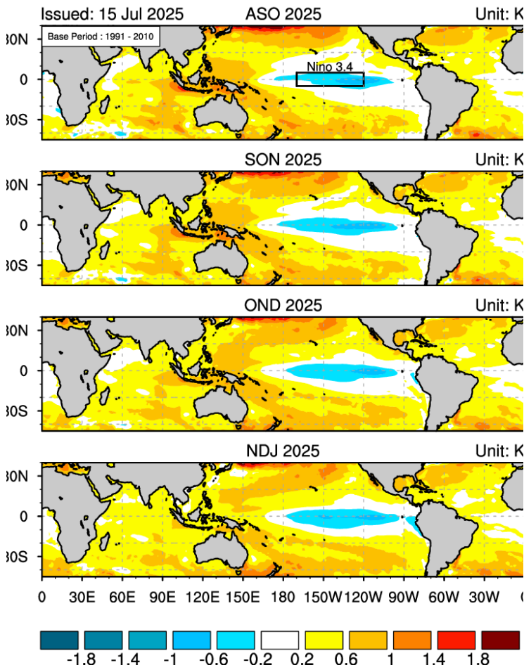
2025년 8월-2026년 1월 해수면온도 평년대비 편차 (평년: 1991-2010)
