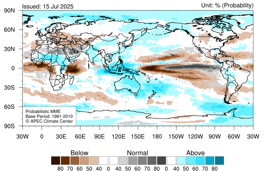
2025년 8월-10월 기온(위)과 강수(아래)의 평년대비 편차 (평년: 1991-2010)
