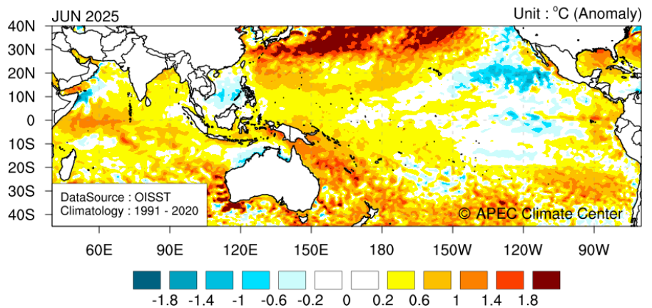
2025년 6월 해수면온도 분포 및 평년대비 편차(평년: 1991-2020)
