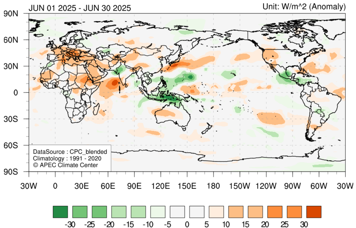
2025년 6월 기온(위) 및 상향장파복사(아래)의 평년대비 편차(평년: 1991-2020)
