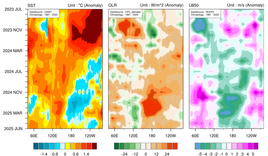
2023년 7월-2025년 6월 해수면온도, 상향장파복사, 850hPa 바람 평년대비 편차의 시간-경도 단면도(평년: 1991-2020)
