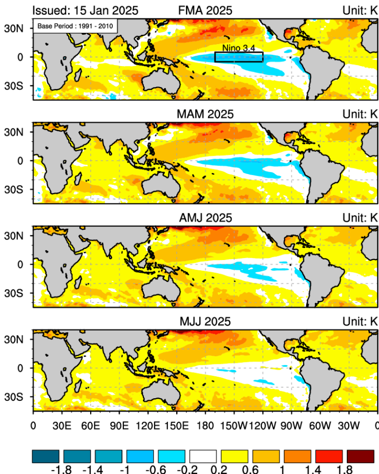
2025년 2월-7월 해수면온도 평년대비 편차 (평년: 1991-2010)
