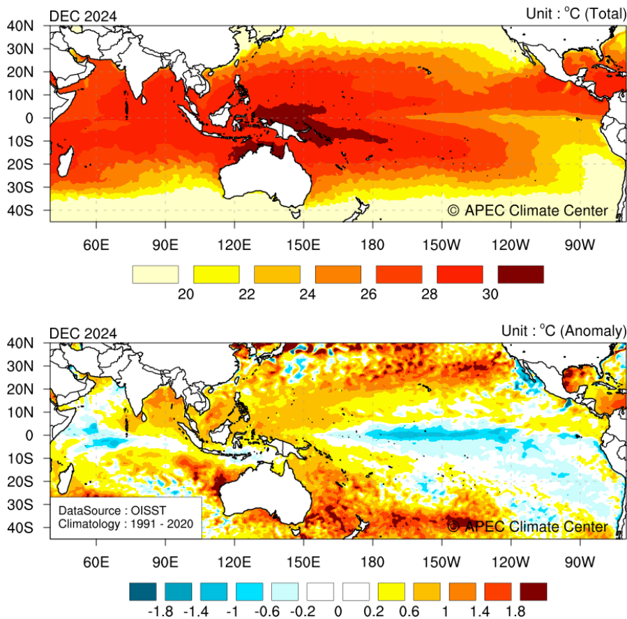
2024년 12월 해수면온도 분포 및 평년대비 편차(평년: 1991-2020)
