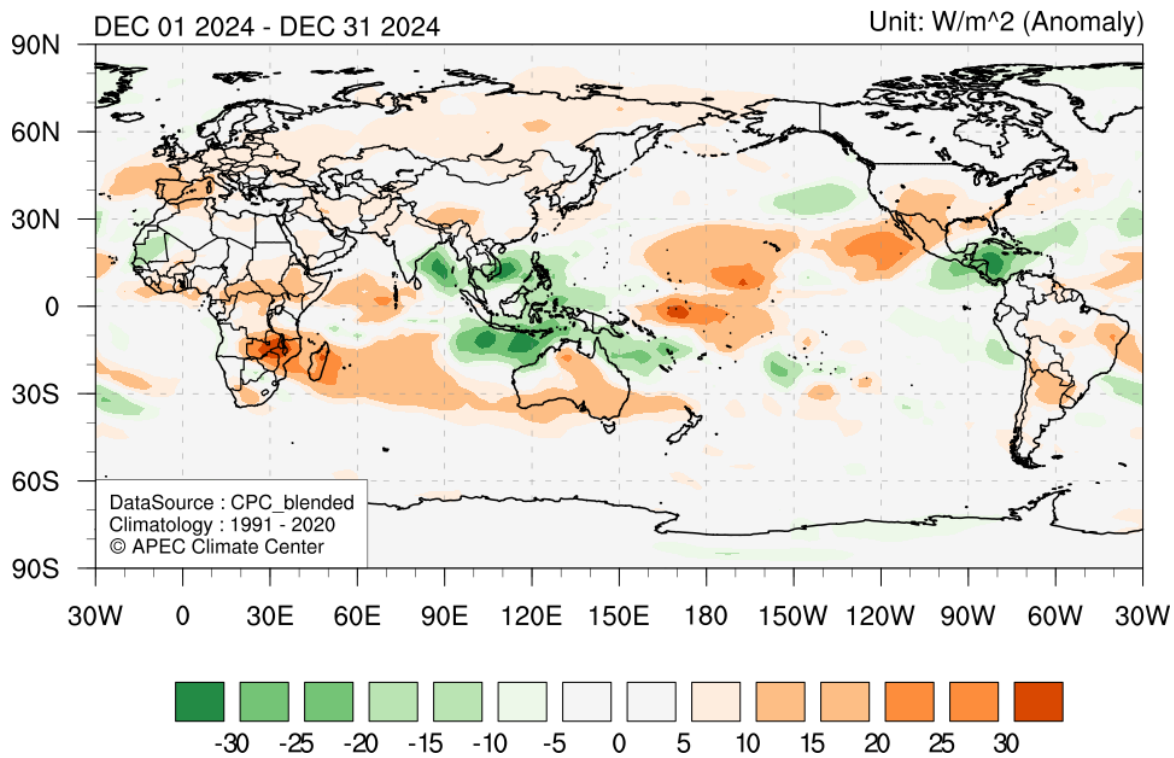
2024년 12월 기온(위) 및 상향장파복사(아래)의 평년대비 편차(평년: 1991-2020)
