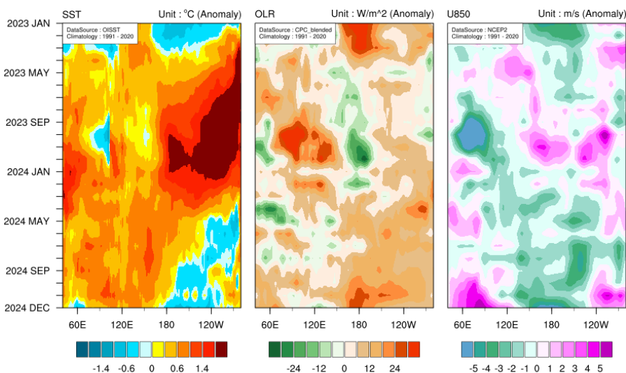
2023년 1월-2024년 12월 해수면온도, 상향장파복사, 850hPa 바람 평년 대비 편차의 시간-경도 단면도(평년: 1991-2020)
