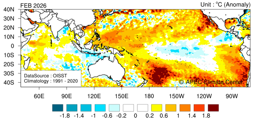
2026 2월 해수면 온도 분포(위) 및 평년대비 편차(아래) (평년: 1991-2020)
