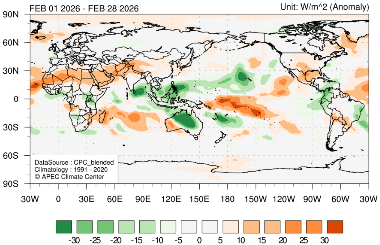
2026 2월 기온 (위) 및 상향장파복사(아래)의 평년대비 편차 (평년 : 1991-2020)
