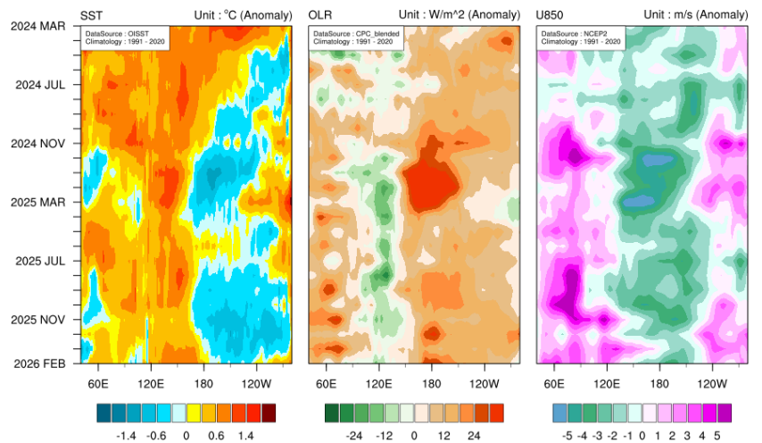
2024 3월 - 2026 2월 적도지역 해수면온도, 상향장파복사, 850hPa 동서 바람 평년대비 편차의 시간-경도 단면도 (평년: 1991- 2020)
