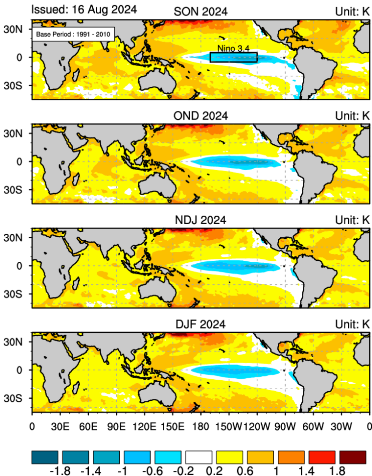
2024년 9월-2025년 2월 해수면온도 평년대비 편차 (평년: 1991-2010)
