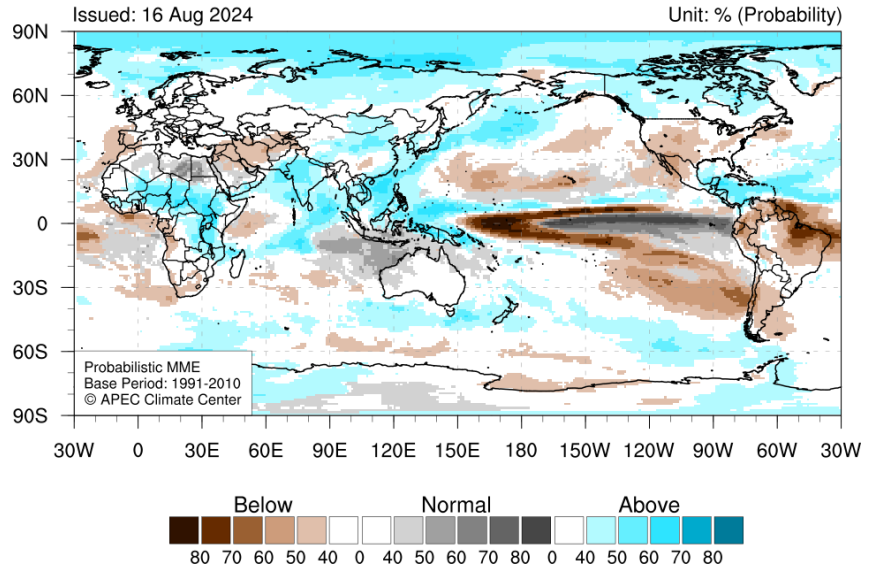
2024년 9월-11월 기온(위)과 강수(아래)의 평년대비 편차 (평년: 1991-2010)
