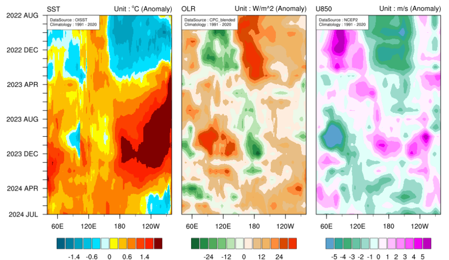
2022년 8월-2024년 7월 해수면온도, 상향장파복사, 850hPa 바람 평년대비 편차의 시간-경도 단면도(평년: 1991-2020)
