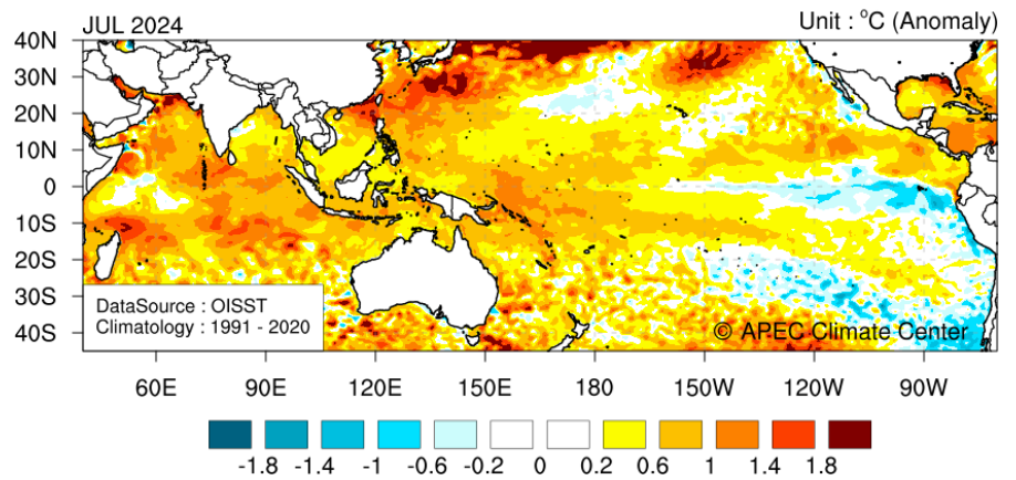
2024년 7월 해수면온도 분포 및 평년대비 편차(평년: 1991-2020)
