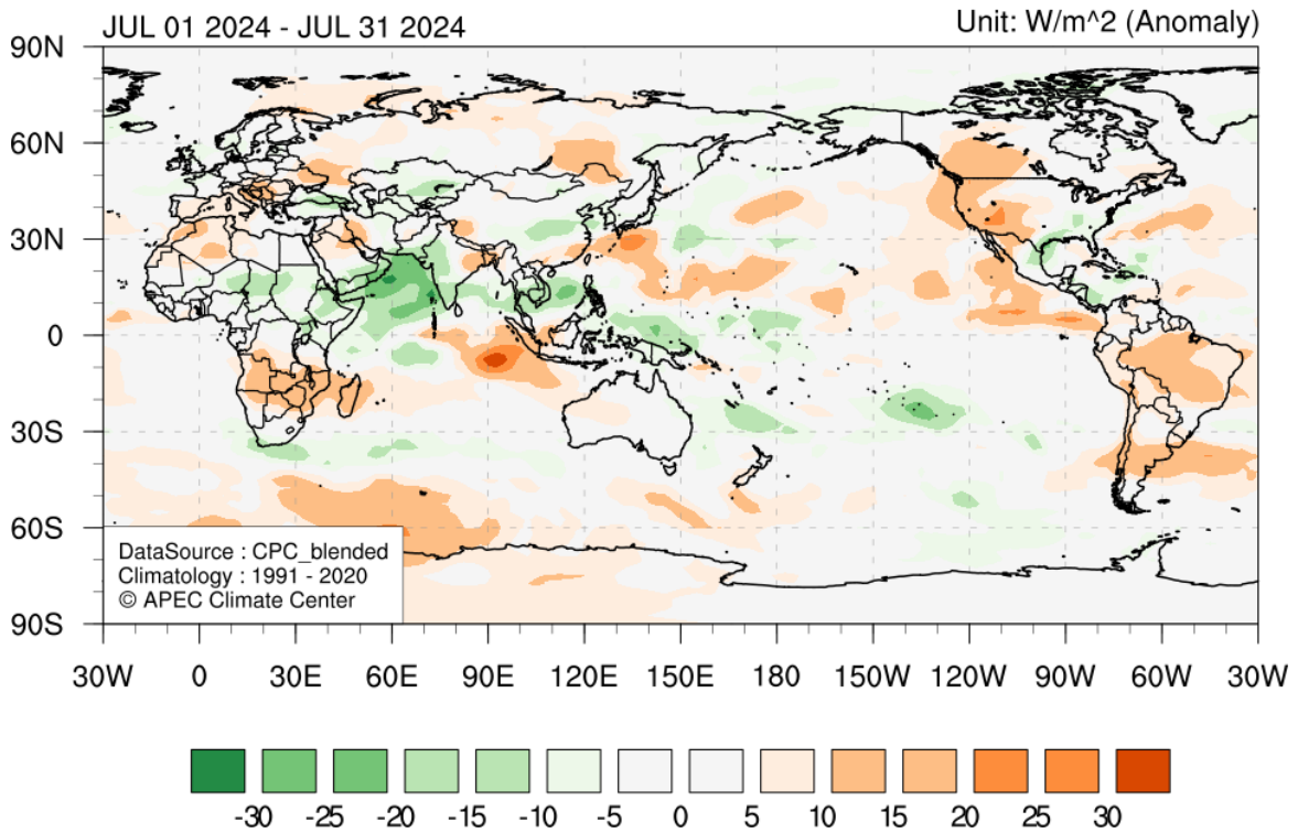
2024년 7월 기온(위) 및 상향장파복사(아래)의 평년대비 편차(평년: 1991-2020)
