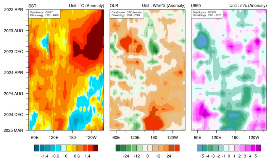
2023년 4월-2025년 3월 해수면온도, 상향장파복사, 850hPa 바람 평년대비 편차의 시간-경도 단면도(평년: 1991-2020)
