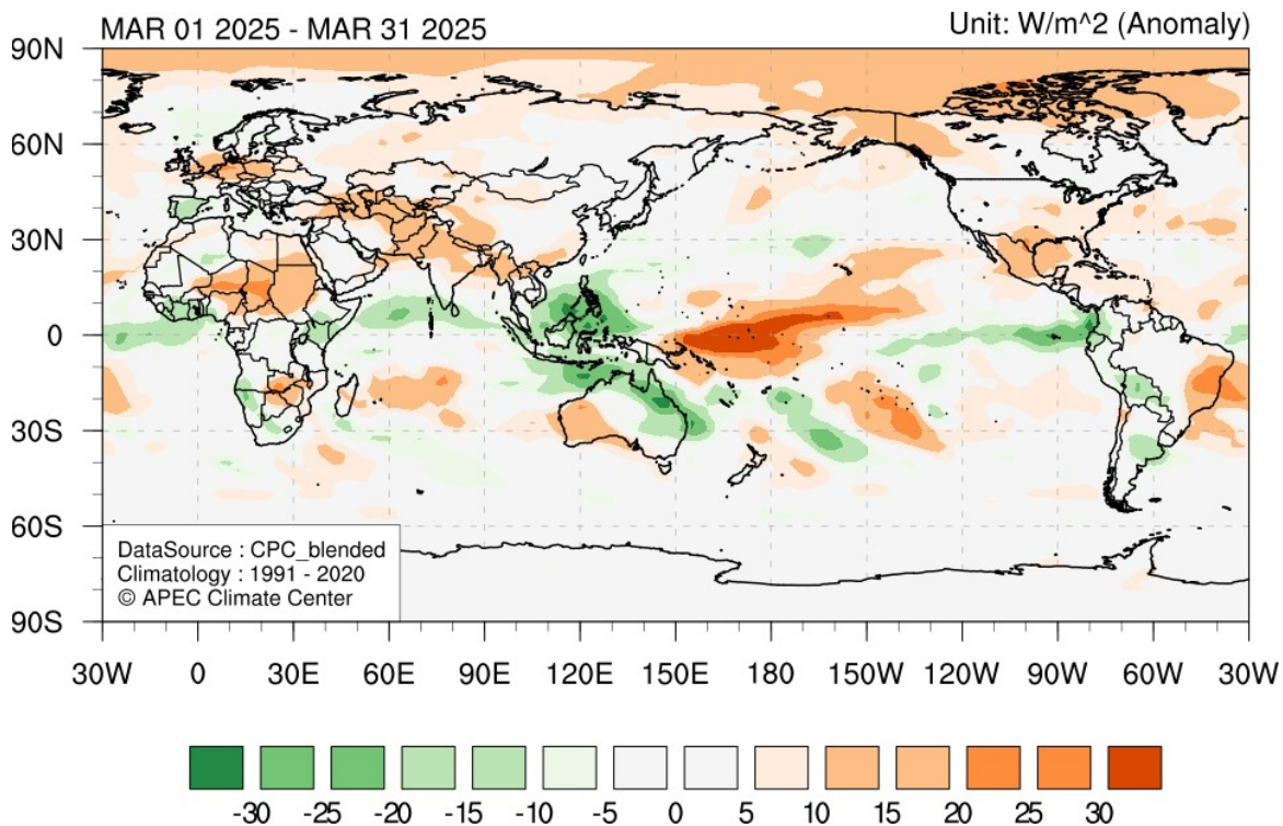
2025년 3월 기온(위) 및 상향장파복사(아래)의 평년대비 편차(평년: 1991-2020)
