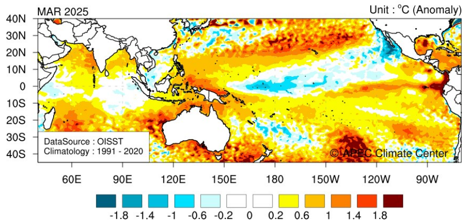
2025년 3월 해수면온도 분포 및 평년대비 편차(평년: 1991-2020)
