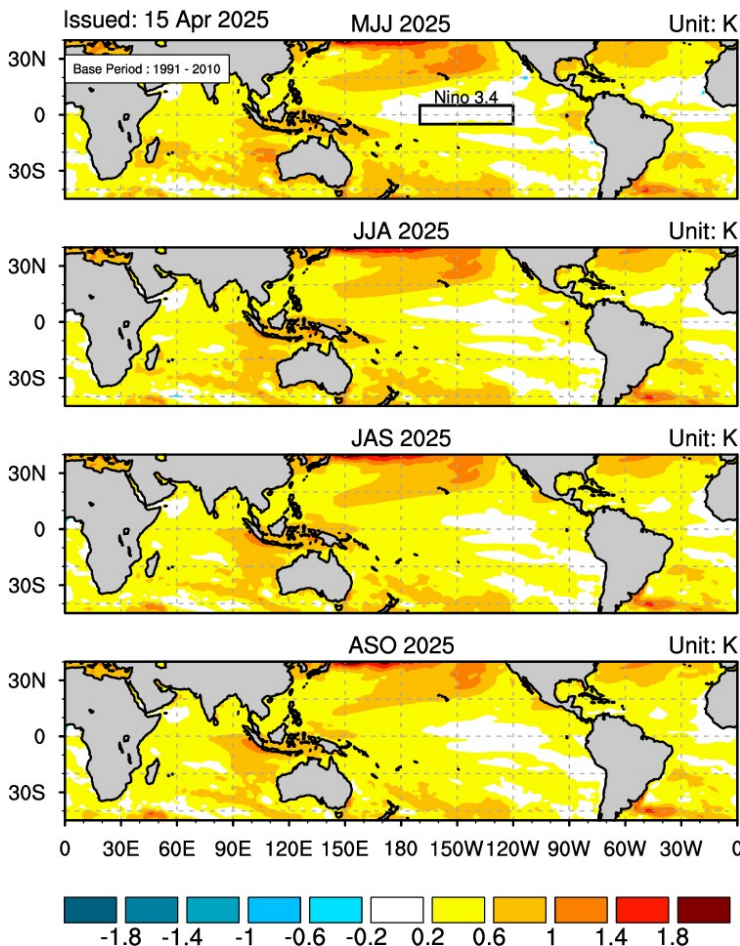
2025년 5월-10월 해수면온도 평년대비 편차 (평년: 1991-2010)
