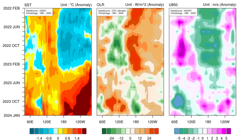
2022년 2월-2024년 1월 해수면온도, 상향장파복사, 850hPa 바람 평년대비 편차의 시간-경도 단면도(평년: 1991-2020)
